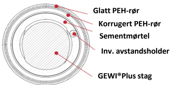
Tversnitt av fri lengden
