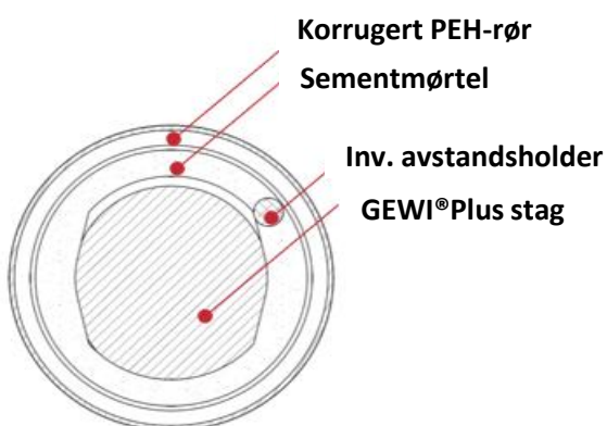
Tversnitt av forankringslengden
